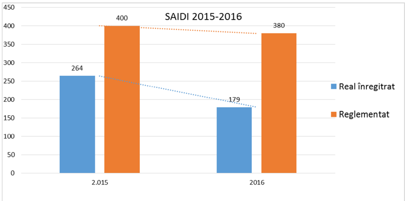
Figura 4.1. Evoluția Indicatorului SAIDI pentru perioada 2015-2016
